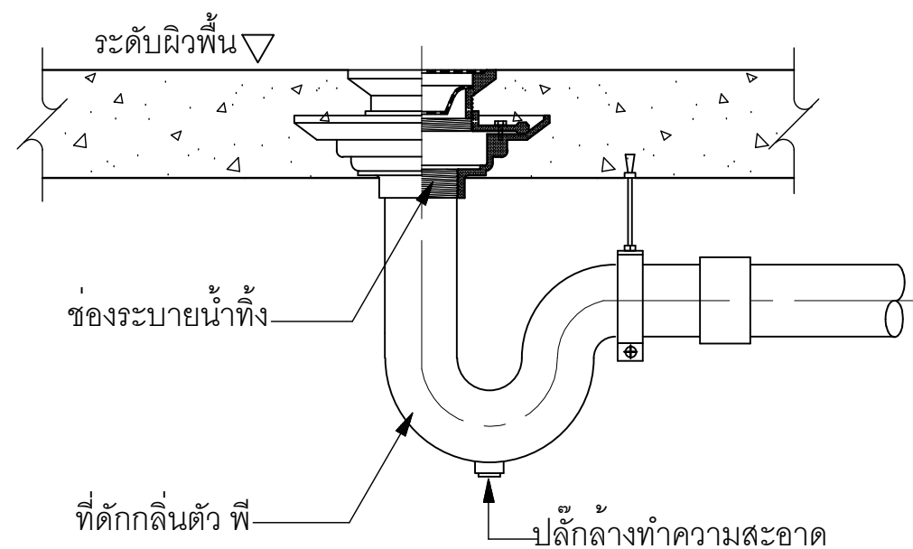
ช่องระบายน้ำทิ้งที่พื้น ( FD )
